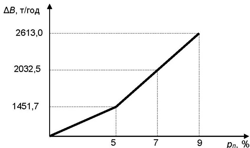
Рис. 1. Зависимость годовой экономии условного топлива \Delta B , т/год от величины непрерывной продувки котла p_p , % (Arial, 11 points)
