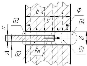
Рис. 2. Картина поля при выходе из зазора магнитопроводящего элемента
