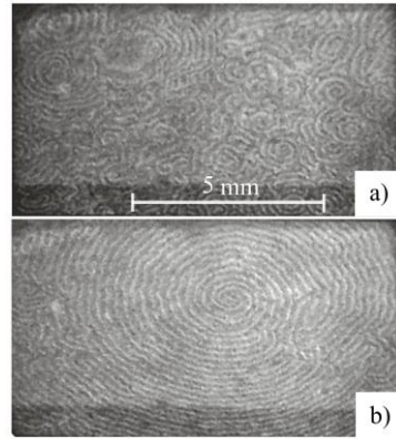
Рис. 5. Спиральные волны: а) – U_{\Pi} = 27 В, б) – U_{\Pi} = 18 В
