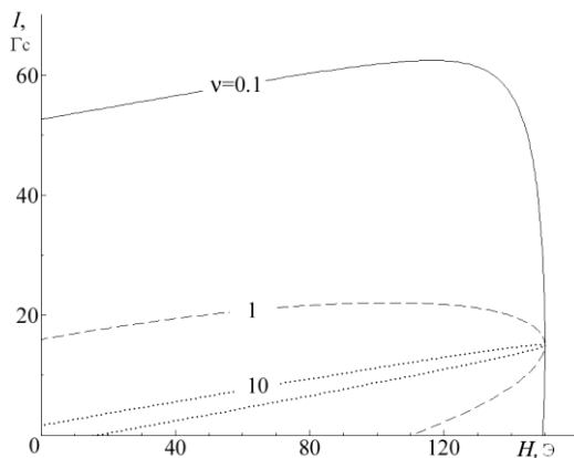
Рис. 3. Петли динамической намагниченности суспензии кластеров для H_0 = 150 Э, \mu = 0.11 и различных безразмерных частот \nu_c
