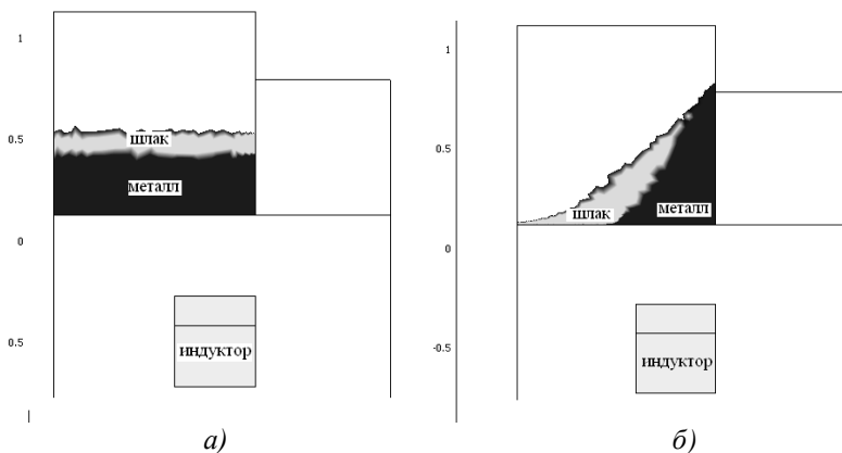
Рис.2. Уровень металла в ванне ПА
