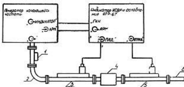
Рис. 3. Схема установки для измерения коэффициентов отражения и ослабления: 1 - аттенуатор, 2 - волноводный тракт, 3 и 5 - направленные ответвители с квадратичными детекторами, 4 - измерительная ячейка, 6 - согласованная нагрузка
