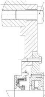
Рис. 8. МЖГ вентилятора ВЦ-25
