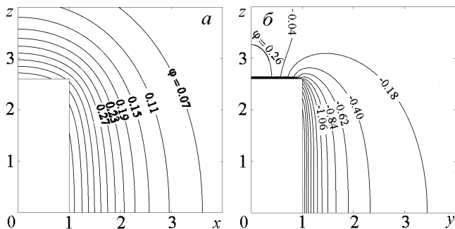
Рис. 3. Эквипотенциальные линии магнитоферретического потенциала \varphi поперечно намагниченного цилиндра (полуудлина цилиндра l=2,6 радиуса, безразмерная напряженность поля P = 1.5 ) a – в плоскости y=0 , b – в плоскости x=0
