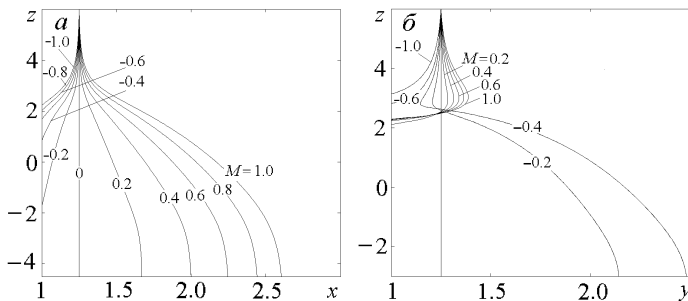
Рис. 2. Траектории частиц, полученные для разных значений магнитоферретического параметра M (прицельное расстояние \delta = 1.25 , полуудлина цилиндра 2.6 радиуса, безразмерная напряженность поля P = 1.5 ) a – в плоскости y=0 , b – в плоскости x=0
