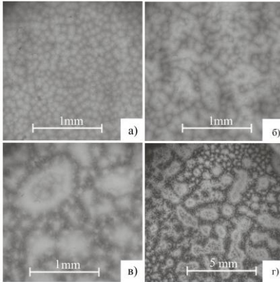
Рис. 4. Структурные образования в слое коллоида при воздействии заданного тока и постоянном напряжении на электродах ячейки U_{\Pi} : а – U_{\Pi} = 9 В, б – U_{\Pi} = 12 В, в – U_{\Pi} = 17 В, г – U_{\Pi} = 22 В
