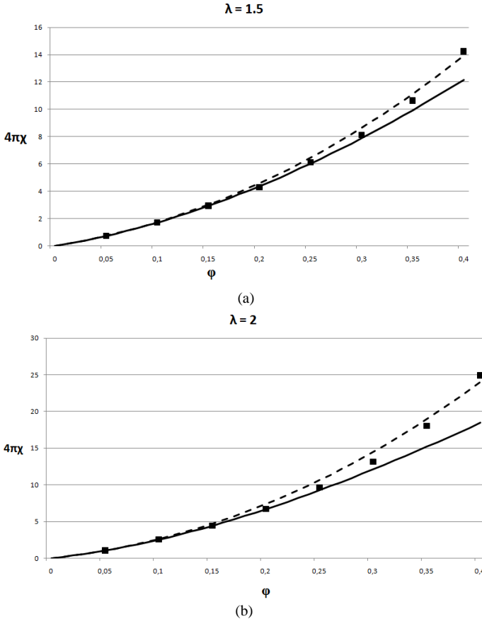
Рис. 3. Начальная магнитная восприимчивость в зависимости от объёмной концентрации феррочастиц \phi . (а): \lambda = 1.5 (b): \lambda = 2 . Сплошная линия соответствует формуле (2), пунктирная линия – формула (1), точки – результаты компьютерного моделирования
