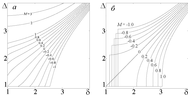
Рис. 4. Функция расстояния выхода от прицельного расстояния при разных значениях магнитоферретического параметра M a – в плоскости y=0 , b – в плоскости x=0
