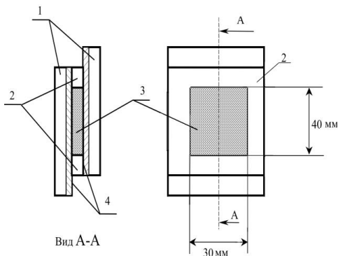
Рис. 1. Конструкция ячейки: 1 – стеклянные пластины, 2 – прокладка из фторопласта, 3 – слой МЖ, 4 – прозрачные электроды из \text{In}_2\text{O}_5\text{:SnO}_2
